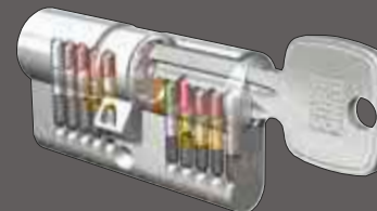
STANDARD - PROFILZYLINDER
